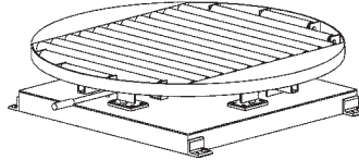
G-621 Tilt Table
