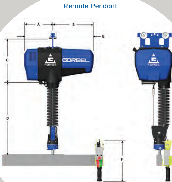
Remote Pendant
